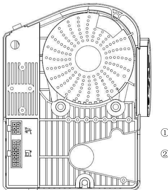
Рис 1. A2 – разъёмы блока управления
